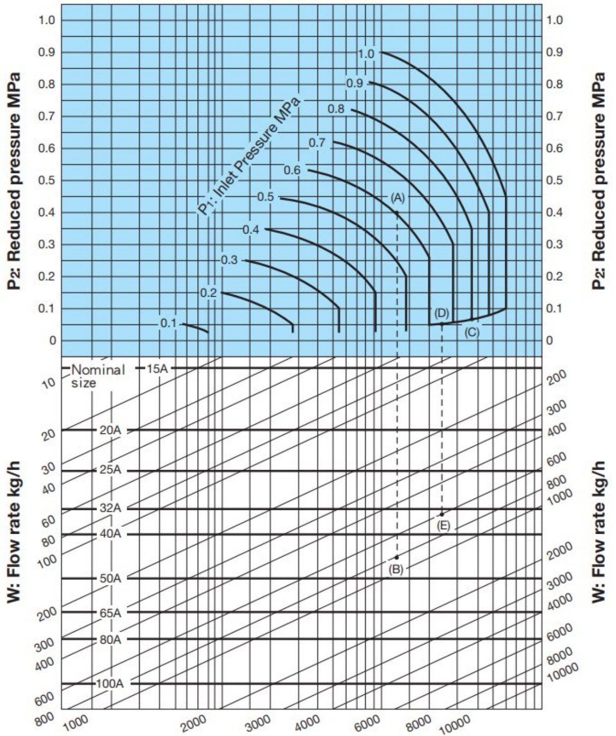
Диаграмма подбора номинального размера (для пара)
