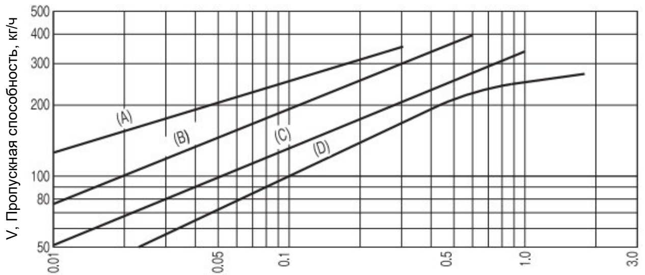
График производительности*
