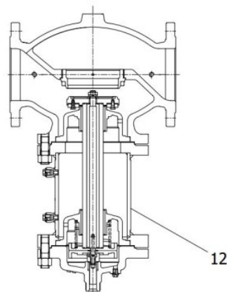
DN150-DN200 (с удлинителем штока)
